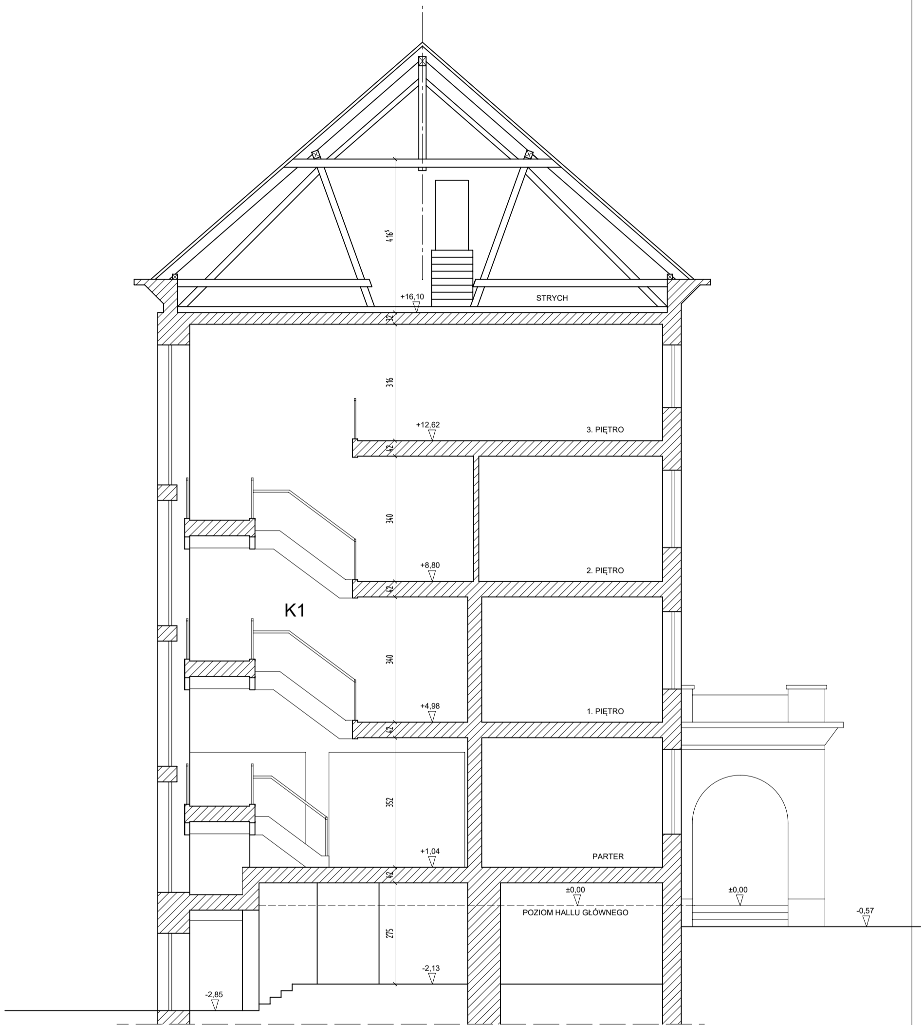
PRZEKRÓJ B-B
