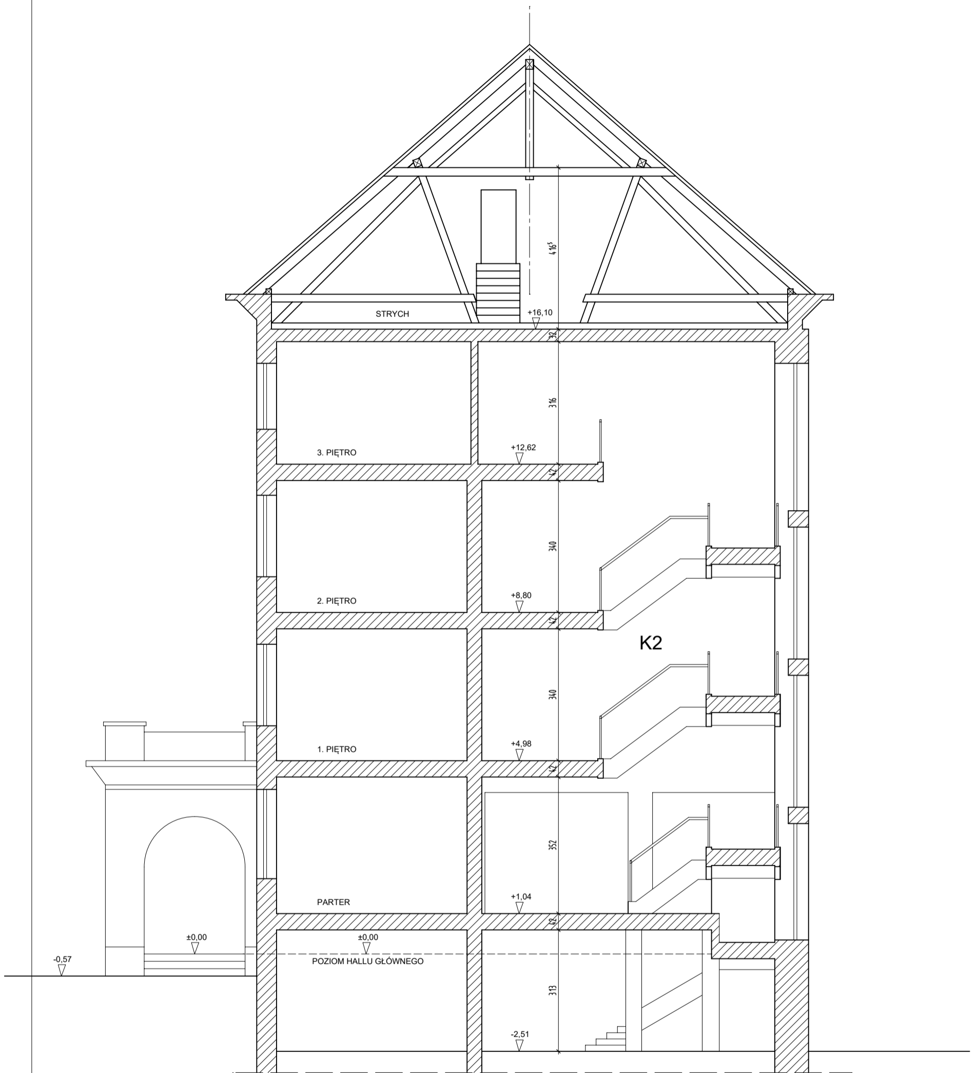
PRZEKRÓJ A-A
