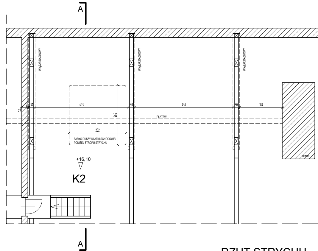
RZUT STRYCHU
