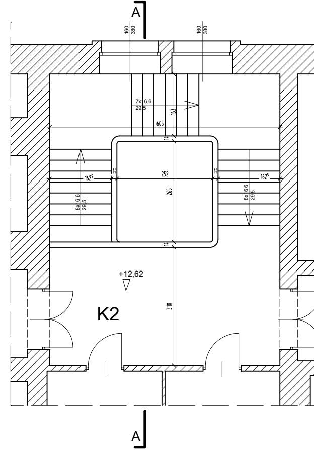
RZUT 3 PIĘTRA
