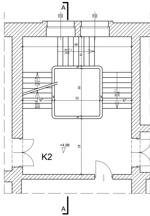
RZUT 1. PIĘTRA
