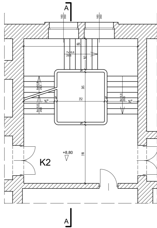
RZUT 2. PIĘTRA
