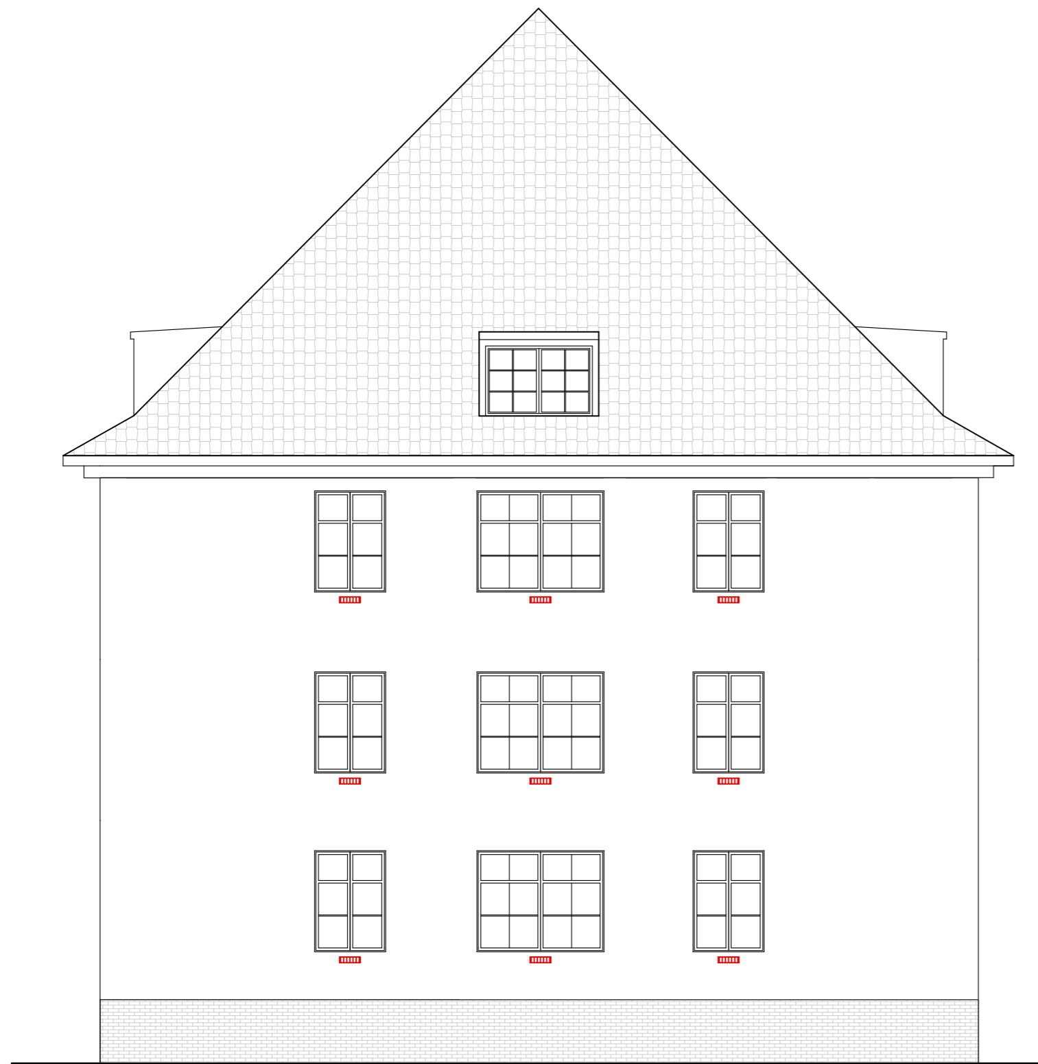
ELEWACJA WSCHODNIA
