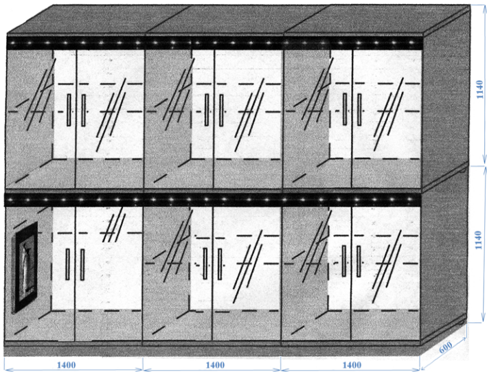
Rysunek poglądowy gablot szklanych
